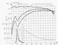
Рис. 69. Характер процесса сушки конденсаторов с бумажным диэлектриком:
