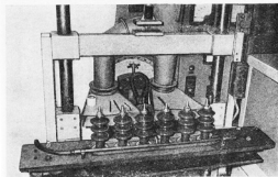
Рис. 45. Рабочий стол для высокочастотной припайки арматуры
