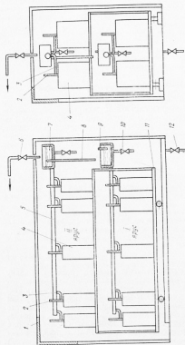
Рис. 67. Схема индивидуальной заливки конденсаторов:
