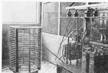
Рис. 91. Дроссели, применяемый в установках переменного тока повышенной частоты
