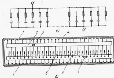
Рис. 40. Электрическая схема соединения (а) и схема пайки токоподводов (б) при параллельном соединении секций в пакете (конденсатор КС0.66 однофазный): 1 — секция, 2 — соединительная шина, 3 — место для припайки отвода, 4 — корпусная изоляция, 5 — предохранитель, 6 — токоподвод, 7 — межсекционная прокладка
