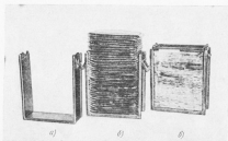
Рис. 37. Сборка пакетов конденсатора ЭСВ: а — струбина, б — колонка секций в струбине, в — пакет после запрессовки
