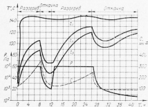
Рис. 70. Характер процесса предварительной сушки конденсаторов:
