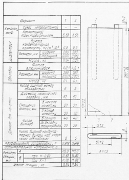
Рис. 32. Чертеж и технические данные секции конденсатора КС2-6,3-75-2У3:
