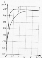
Рис. 73. Зависимости емкости от времени пропитки конденсаторным маслом конденсаторов из бумаги: 1 — КОИ-1, 2 — КОИ-2
