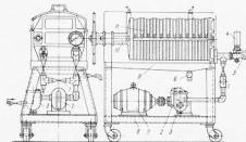
Рис. 80. Фильтр-пресс
