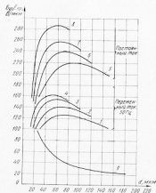
Рис. 26. Зависимости напряженности возникновения частичных разрядов (кривая 9) и электрической прочности от толщины бумажно-масляного диэлектрика между обкладками конденсатора из бумаги КОИ-2 толщиной:
