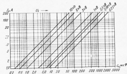
Рис. 94. Номограмма для выбора предела измерения по току
