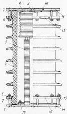
Рис. 74. Устройство конденсатора ДМР80-0,0044:
