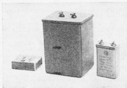
Рис. 25. Конденсаторы для люминесцентных светильников
