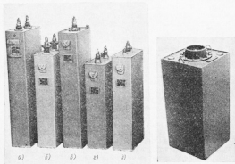
Рис. 18. Импульсные конденсаторы: а — ИК6-200ХТ2, б — ИК6-5-58У4, в — ИК25-140У4, г — ИК25-6-140У4, д — ИК6-120У4
