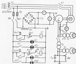
Рис. 92. Схема установки переменного тока повышенной частоты
