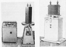
Рис. 96. Стенды для испытания конденсаторов: а — на вибропрочность, б — на ударную прочность
