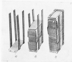
Рис. 36. Сборка пакетов конденсатора СМ166/1/3-14У1: а — скрепляющие планки с нижней щекой, б — колонка секций, в — пакет после запрессовки
