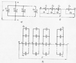
Рис. 2. Соединение секций конденсаторов:
