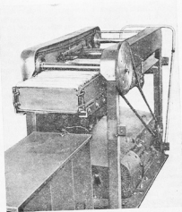
Рис. 42. Станок для механического облуживания торцов пакетов конденсаторов ЭСВ
