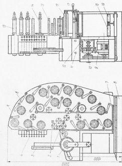
Рис. 19. Устройство намоточного станка SHK-18
