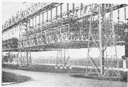
Рис. 13. Конденсаторная батарея на Михайловской преобразовательной подстанции ЛЭП
