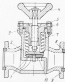
Рис. 64. Устройство сифонного вакуумного клапана
