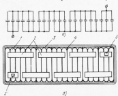
Рис. 39. Электрическая схема соединения (а) и схема пайки токоподводов (б) при смещенном соединении секций в пакете (конденсатор КС6.3): 1 — секция, 2 — перемычка, 3 — корпусная изоляция, 4 — изоляционная прокладка между группами, 5 — место для припайки отводов
