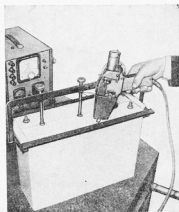
Рис. 48. Приварка крышек конденсаторов в изоляционных корпусах на полуавтомате СА-124М
