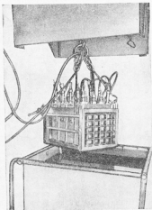
Рис. 50. Стенд для проверки конденсаторов на герметичность воздушным давлением
