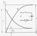
Рис. 3. Заряд конденсатора в цепи постоянного тока
