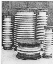
Рис. 16. Конденсаторы связи
