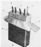
Рис. 41. Пакет конденсатора ЭСВ: а — со стороны охлаждающей трубки, б — со стороны предохранителя; 1 — охлаждающая трубка, 2 — групповой вывод, 3 — обертка, 4 — корпус, 5 — пакет, 6 — предохранитель
