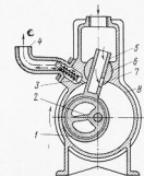
Рис. 56. Устройство золотникового насоса
