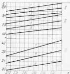
Рис. 28. Зависимости диэлектрической проницаемости бумаги, пропитанной соответственно ТХД (I), касторовым (II) и конденсаторным (III) маслами от коэффициента запрессовки при плотности бумаги:
