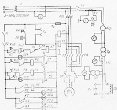
Рис. 87. Схема испытательной установки однофазного переменного тока
